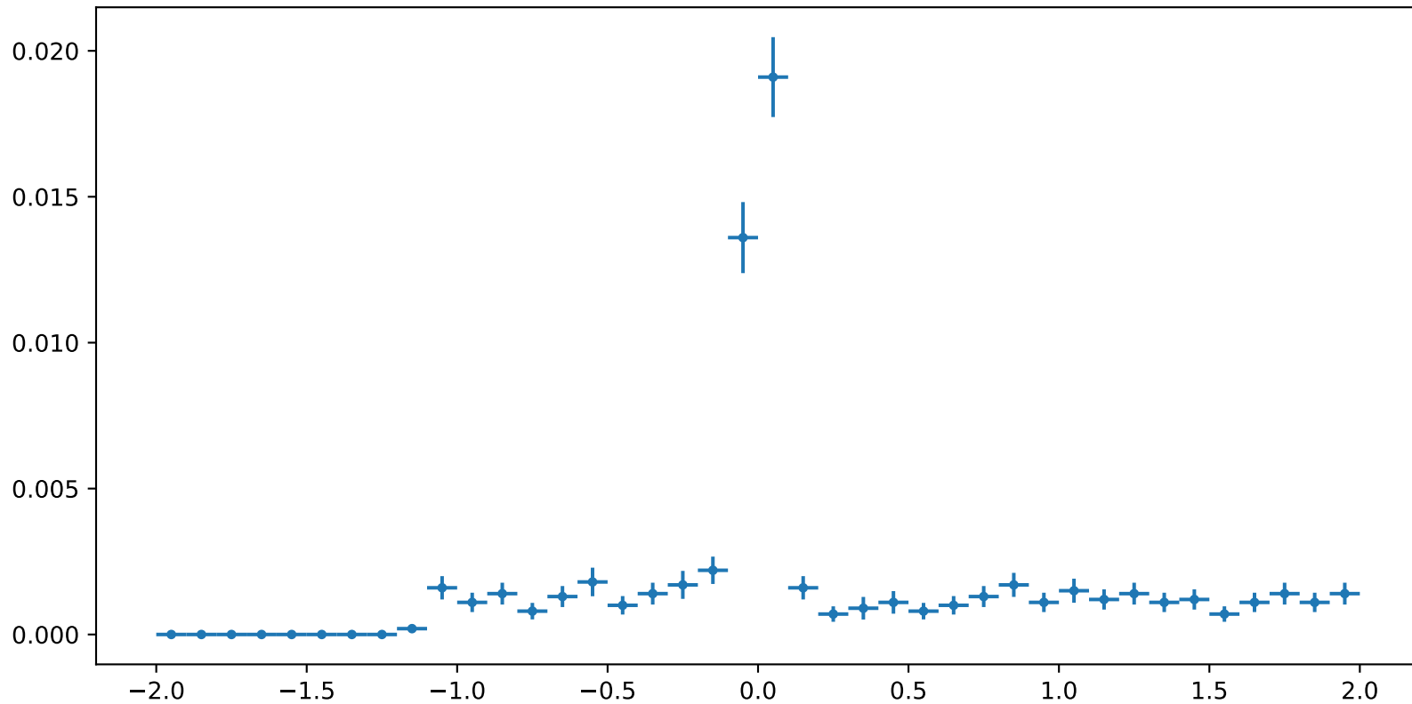
XElectrons
